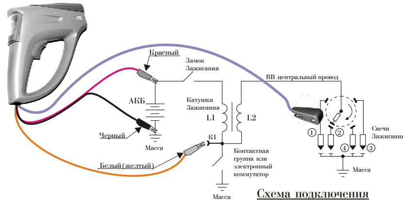
Схема подключения
